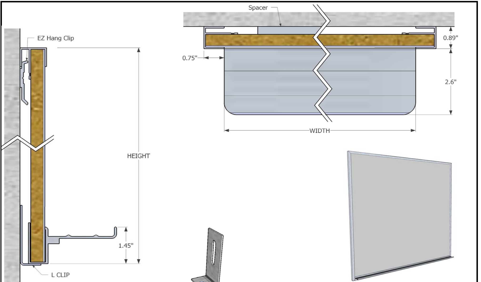
Bottom L-CLIP
